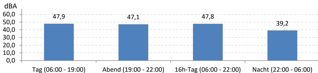
Abb. 7: LEQ bei Pistenbetriebsrichtung "westliche Winde" 327 Stunden im Messzeitraum
